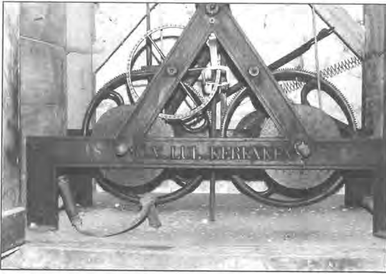
Mechanisme van het torenuurwerk in de kerk van Aalgem.
