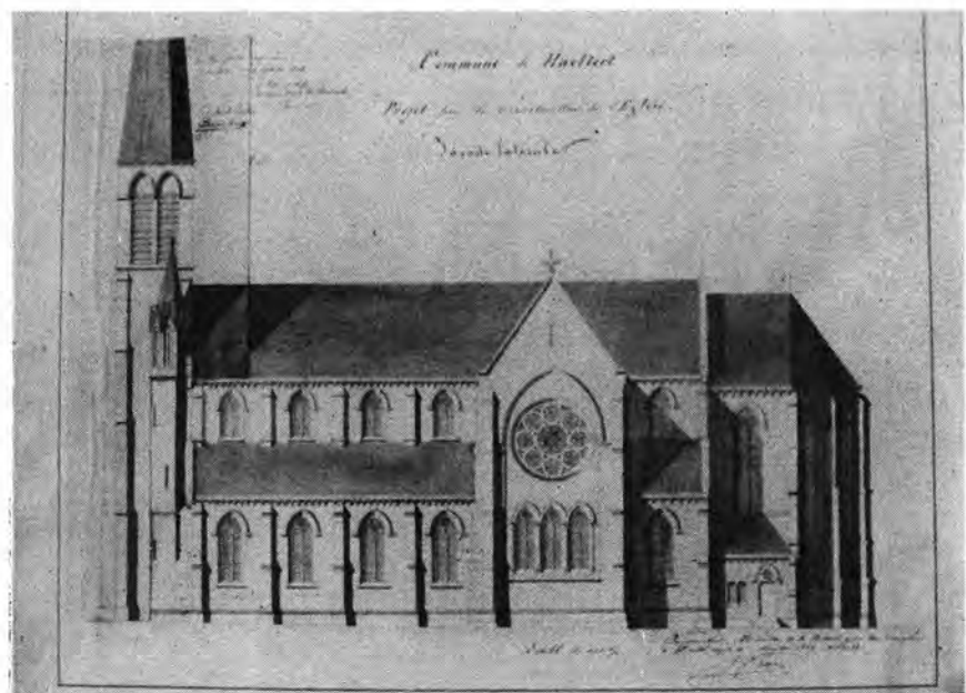
Afb. 15 — Zijgevel
