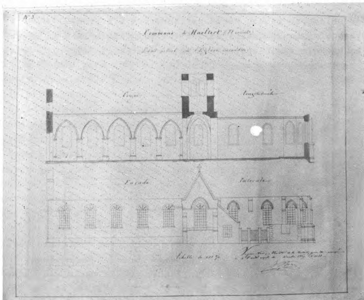
Afb. 4a — De voormalige kapittelkerk, opstandtekening van Ferdinand de Noyette (toestand na de brand)
